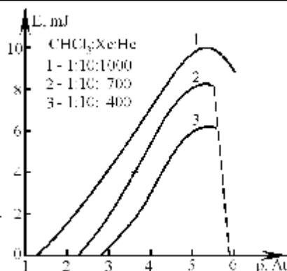
Fig.5. Dependența energiei medii în impuls a laserului XeCl de presiunea absolută a amestecului gazos \text{CHCl}_3 :Xe:He pentru diferite proporții ale componentelor.
