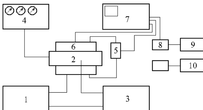
Fig.2. Schema-bloc a instalației experimentale: 1-bloc de alimentare; 2 - camera laser; 3 -sistemul de preionizare; 4 - sistemul de vacuumare și formare a amestecurilor gazoase; 5 - divizor de tensiune înaltă; 6 - sînt pentru măsurarea curentului; 7- osciloscop de tipul C9-4A; 8 - fotocatod FĂC-19; 9 - bloc de alimentare a fotocatodului; 10 - aparat de măsurare a energiei IMO-2M.
