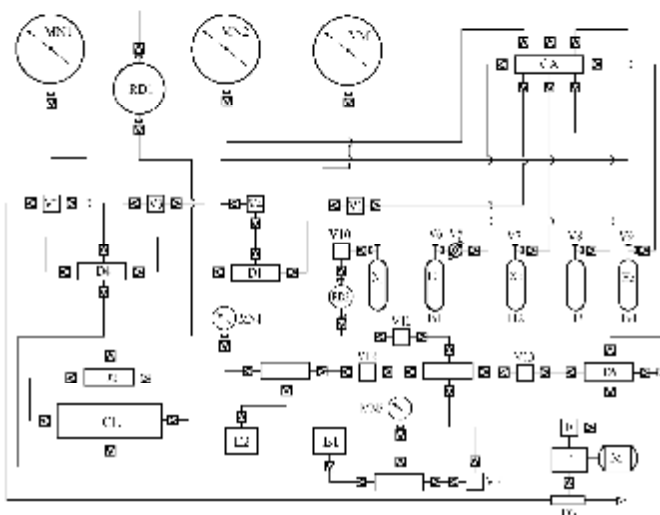
Fig.3. Sistemul de vacuumare și formare a mixturilor gazoase.
