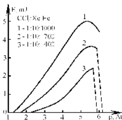
Fig.6. Dependența energiei medii în impuls a laserului XeCl de presiunea absolută a amestecului gazos \text{CCl}_4 :Xe:He pentru diferite proporții ale componentelor.
